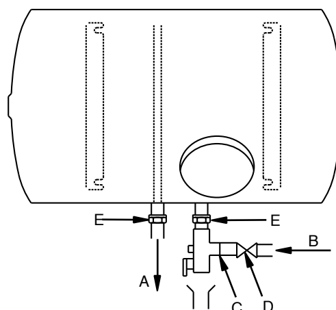
Abbildung 10 - Horizontales Gerät /am Gehäusering
