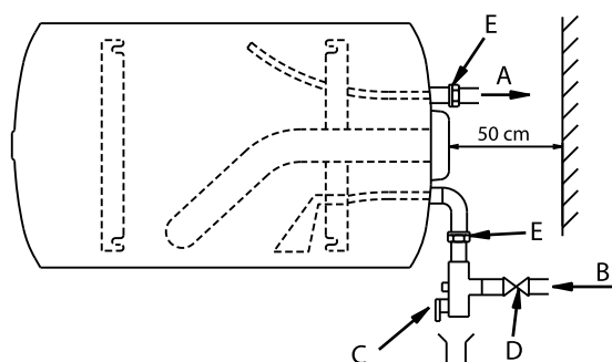
Abbildung 7 - Horizontales Gerät /am Schutzelement – Zuleitungsrohre rechts
