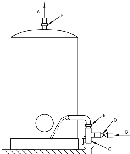
Abbildung 12 - Geräte auf Sockel
