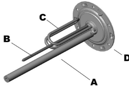
Abbildung 1 - Tauchwiderstand + Magnesiumanode
