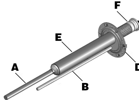
Abbildung 2 - Steatit-Heizwiderstand + Magnesiumanode
